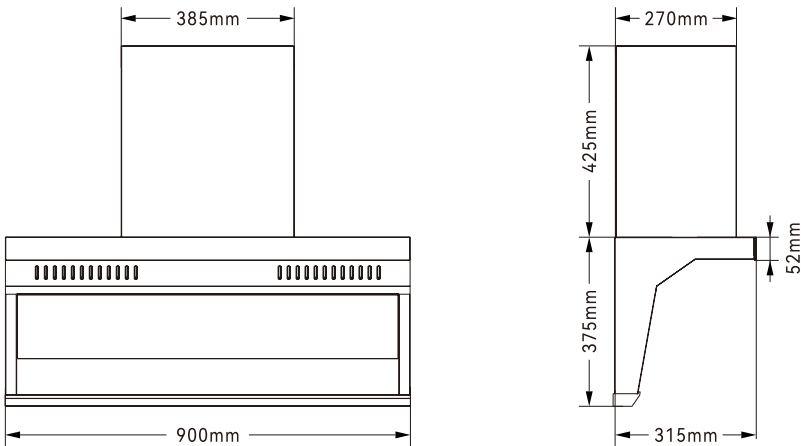
产品型号：CXW-400-BA32BL
