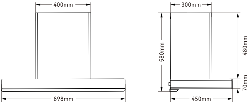
产品型号：CXW-400-BD36BL
