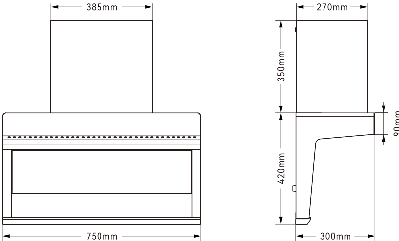
产品型号：CXW-400-BA50BL
