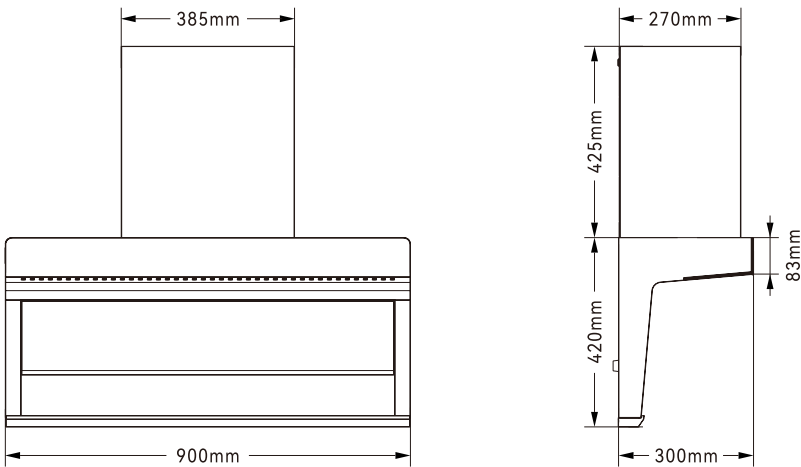
产品型号：CXW-400-BA29BL
